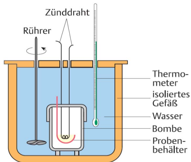
5.1 Ein Bombenkalorimeter
